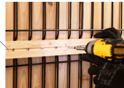
SCHROEFGELEIDER
